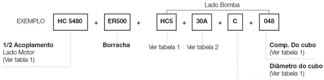
CÓDIGO DE USINAGEM – LADO BOMBA
