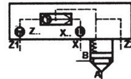
Válvula alternativa
