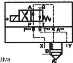
Válvula direccional
