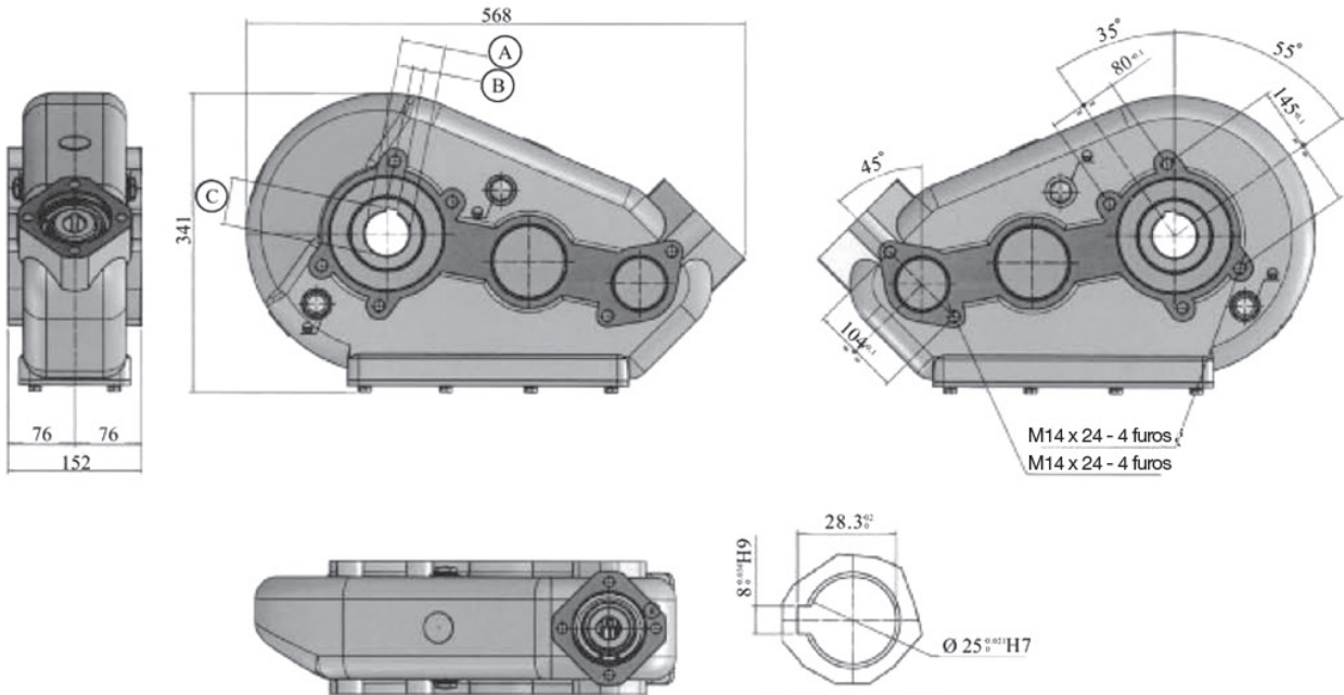
Detalhe A escala 2:1
