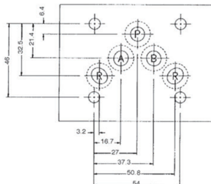
ISO 4401-AC-05-4-A - CETOP 05
