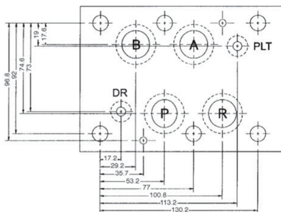
ISO 4401-AE-08-4-A - CETOP 08
