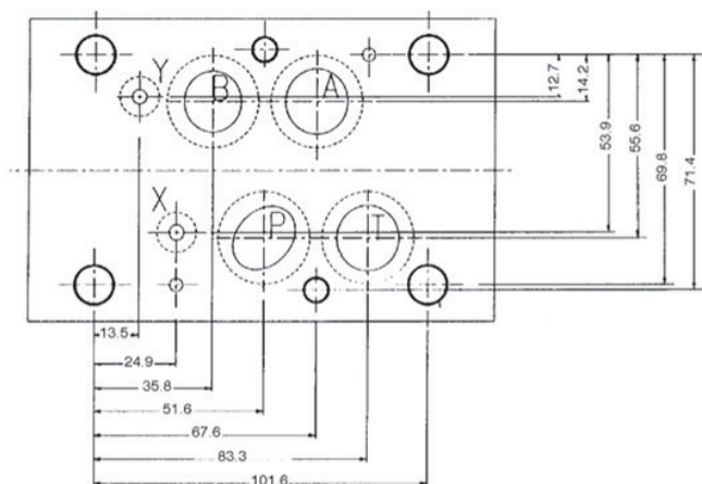
ISO 4401-AD-07-4-A - CETOP 07
